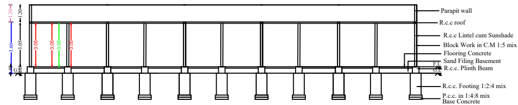
SECTION A-A
