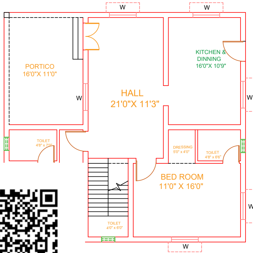
F.F. PLAN
