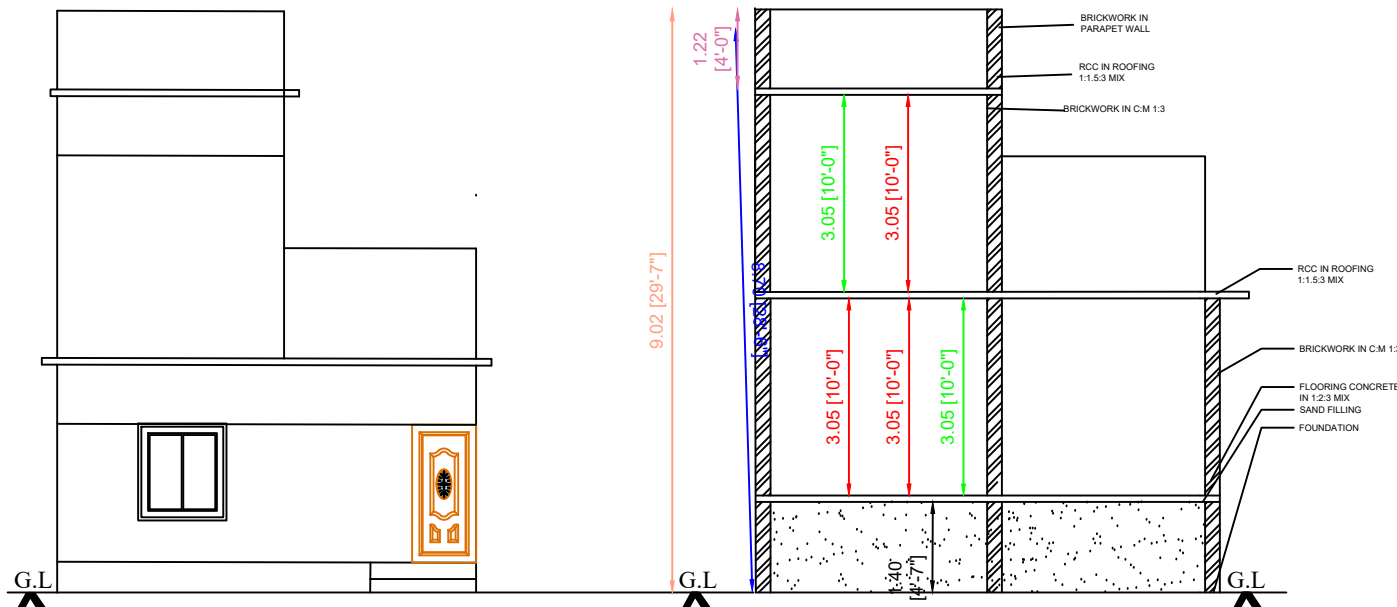
ELEVATION
