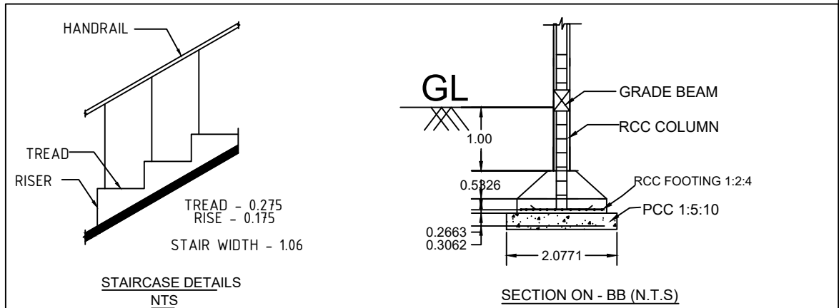
SECTION ON - BB (N.T.S.)
