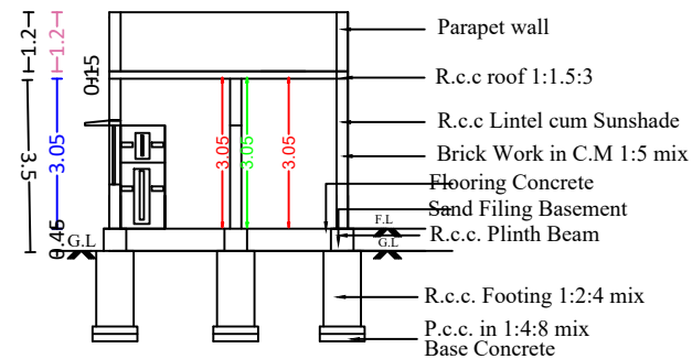
SECTION A-B
