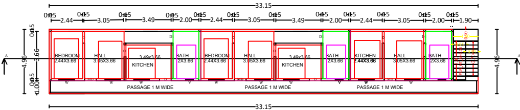
F.F PLAN
