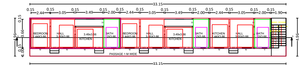
G.F PLAN
