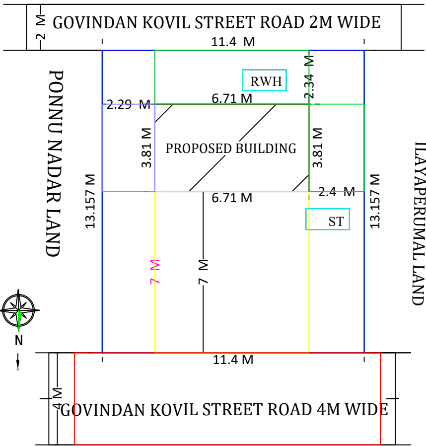
SITE PLAN 1:100 SCALE
