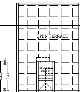
F.F. PLAN
