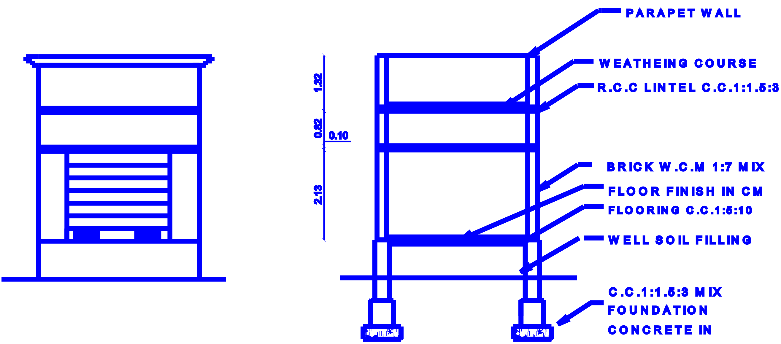
ELEVATION
