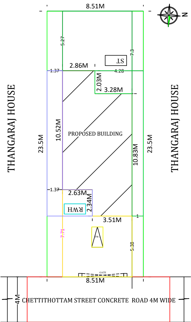
SITE PLAN 1:100 SCALE
