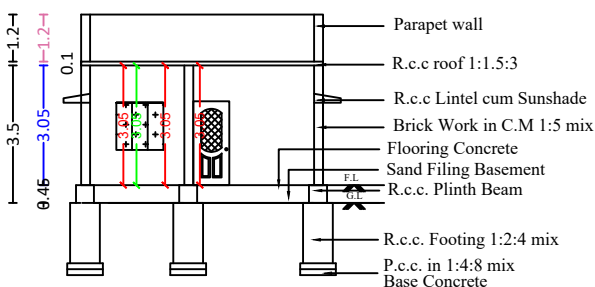
SECTION A-B
