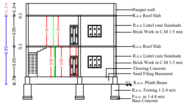
SECTION A-B
