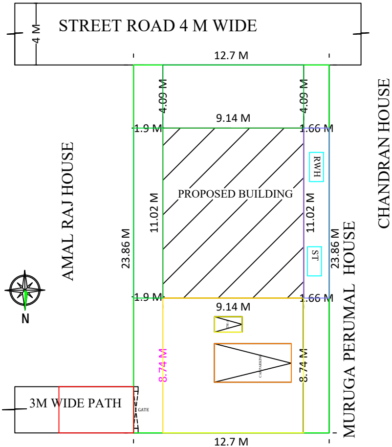
SUR NO 582/7A4 LAND SITE PLAN 1:100 SCALE
