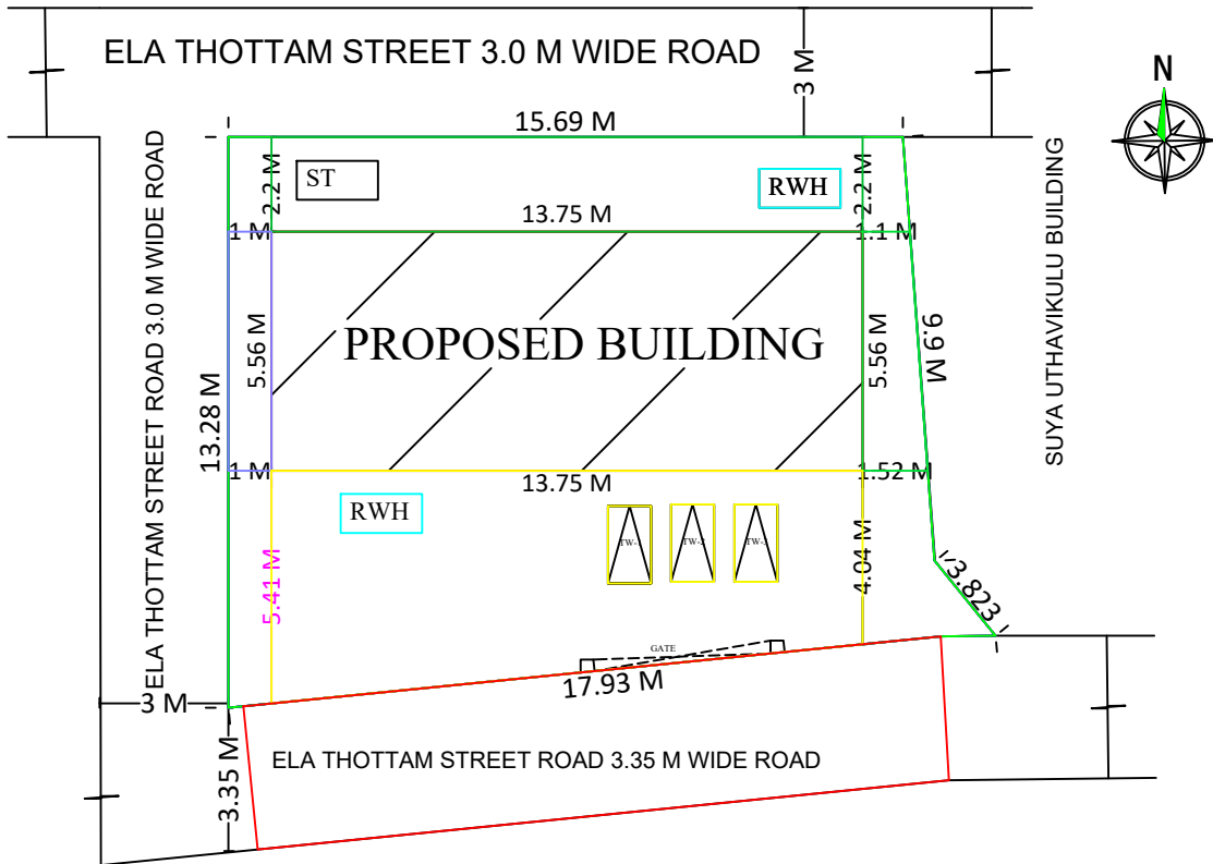
SITE PLAN 1:100 SCALE
