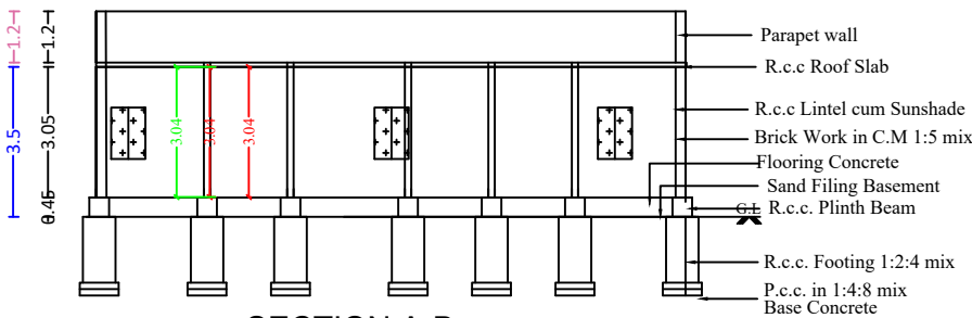
SECTION A-B
