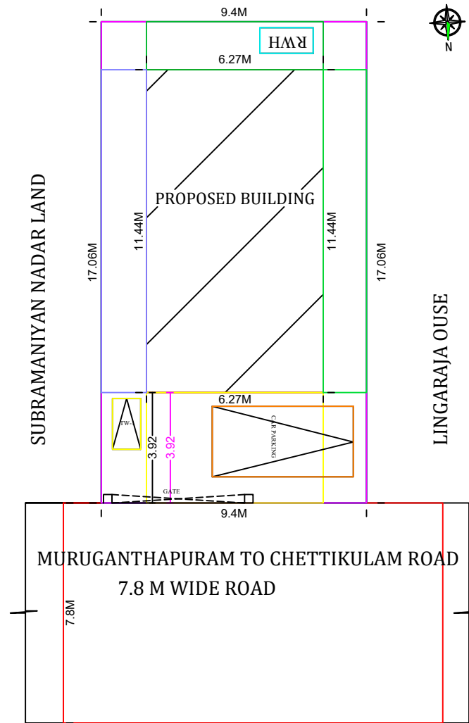
SITE PLAN 1:100 SCALE
