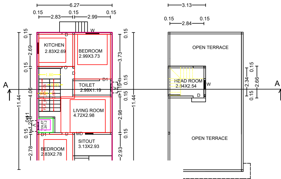
F.F .PLAN
