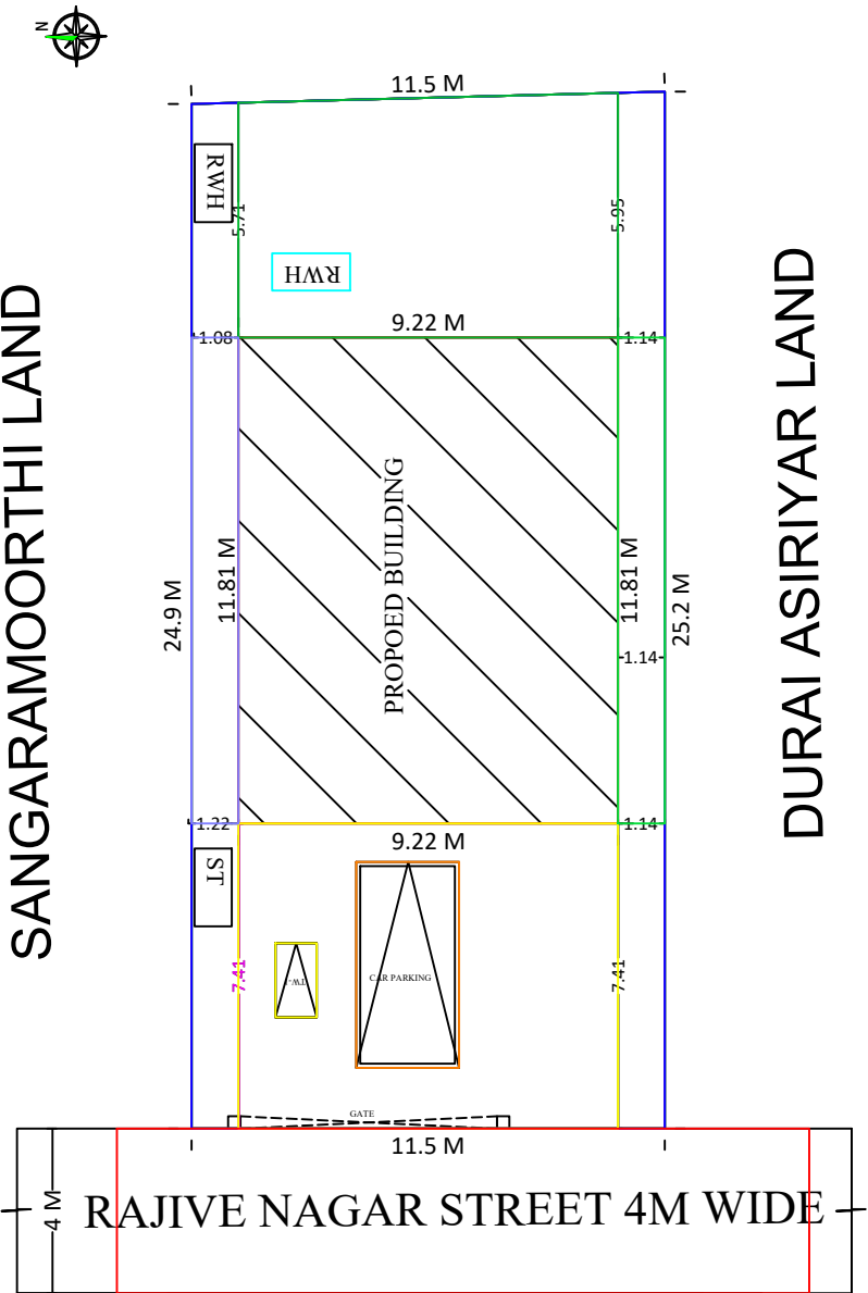
SITE PLAN 1:100 SCALE
