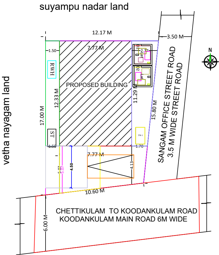
SITE PLAN 1:100 SCALE
