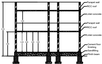
SECTION - AB
