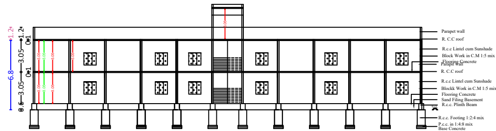
SECTION A-B
