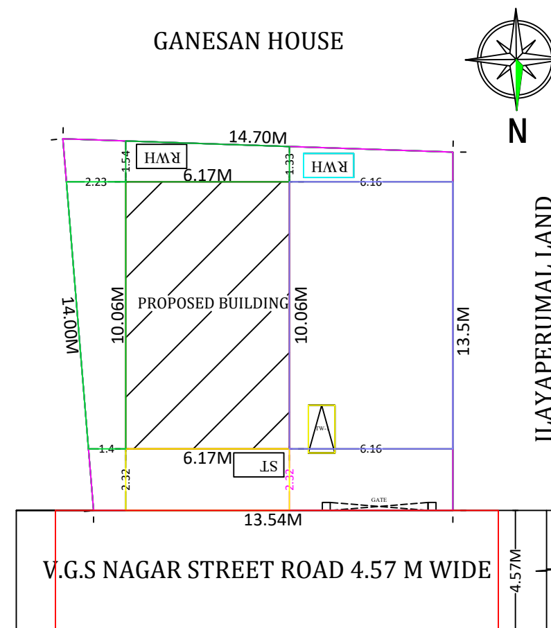
SITE PLAN 1:100 SCALE
