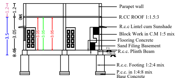
SECTION A-B
