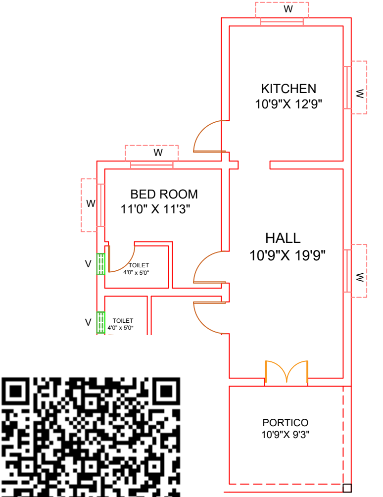
F.F. PLAN
