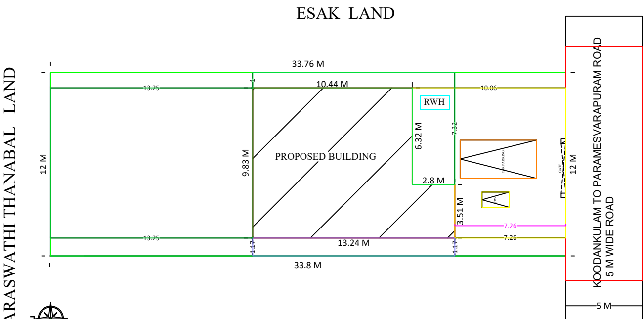
SITE PLAN 1:100 SCALE
