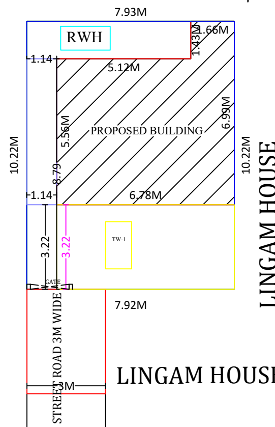
SITE PLAN 1:100
