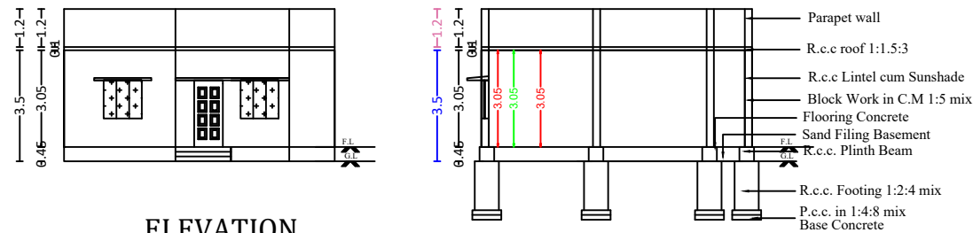
SECTION A-B
