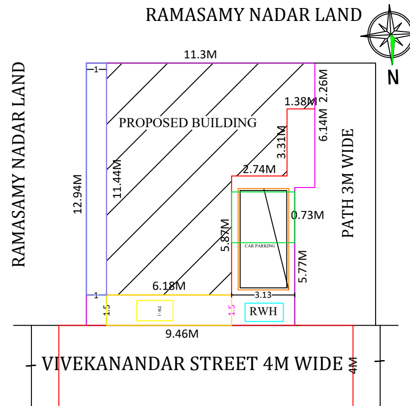
SITE PLAN 1:100
