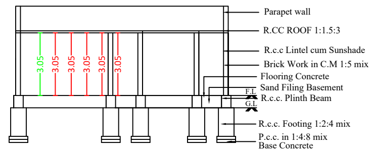
SECTION A-B
