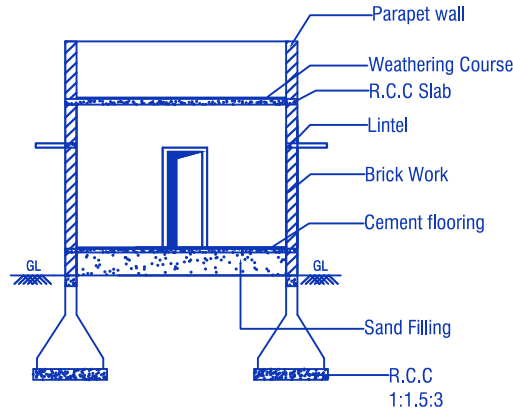
CORSS SECTION ON' AB'
