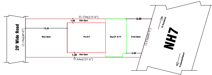
Site Plan (Scale 1:200)
