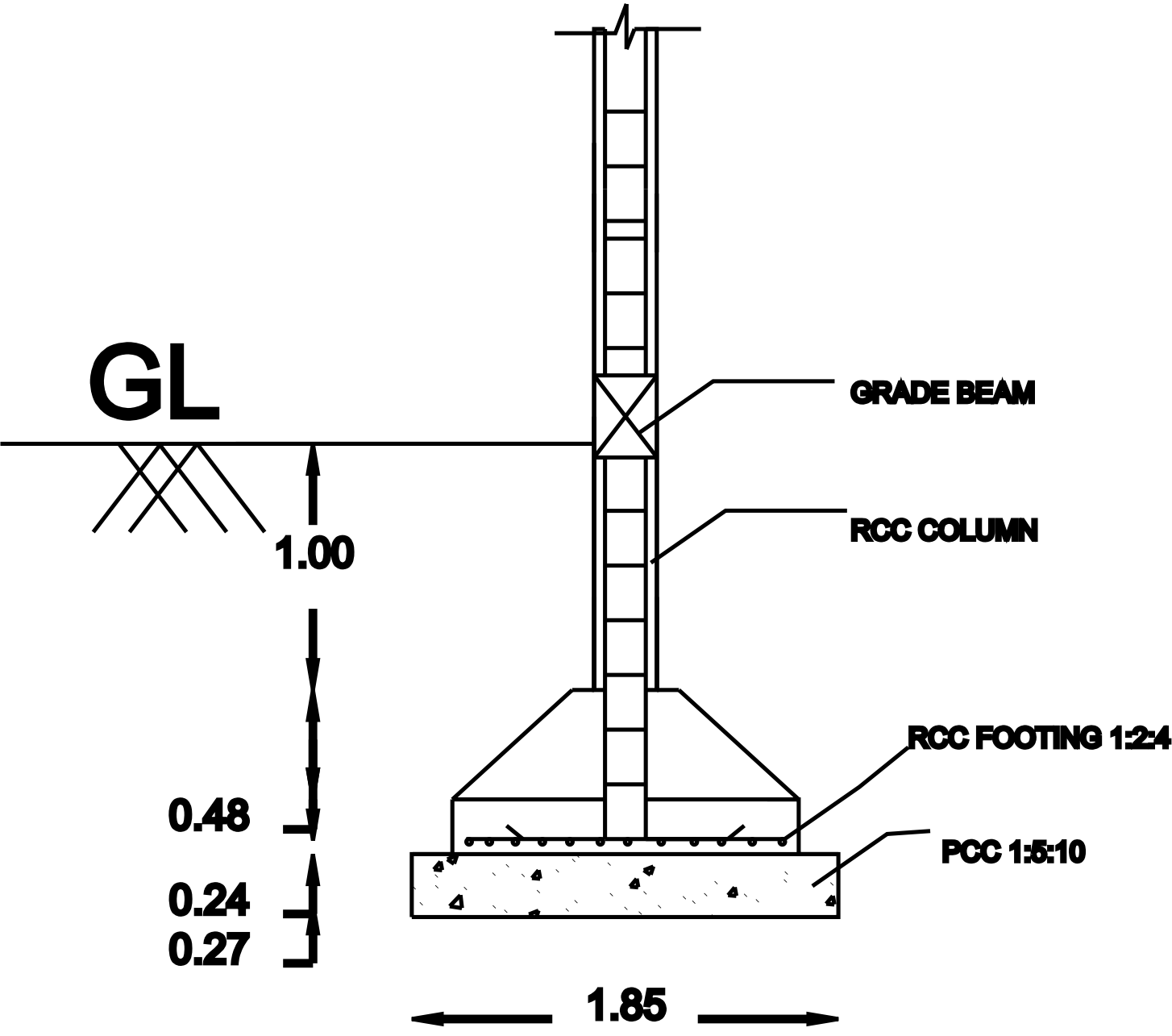
SECTION ON - BB (N.T.S)
