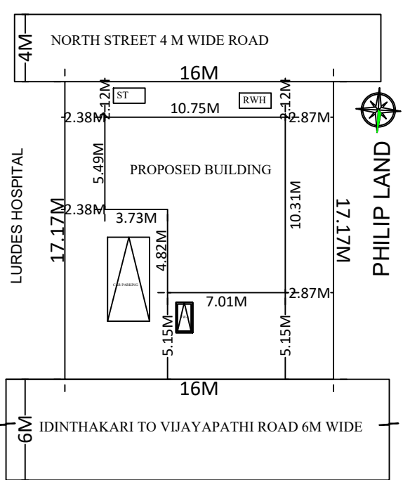
SITE PLAN 1:100 SCALE
