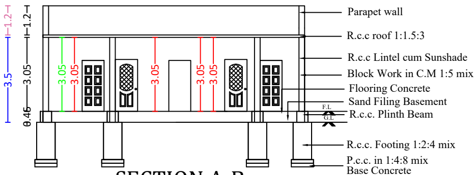
SECTION A-B
