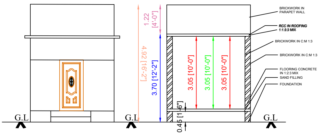
ELEVATION
