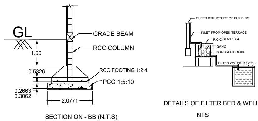
SECTION ON - BB (N.T.S)
