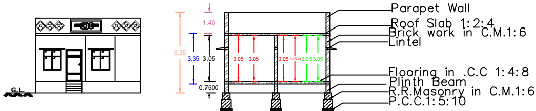
ELEVATION
