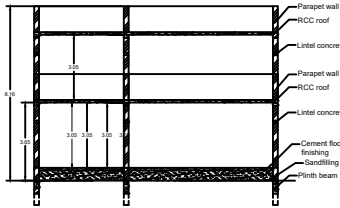
SECTION - AB
