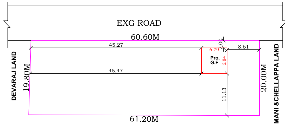
SITE PLAN (SCALE 1:400)
