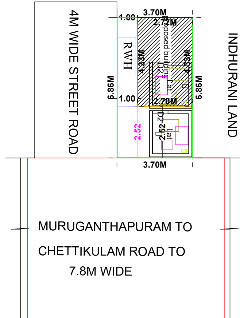
SITE PLAN 1:100 SCALE
