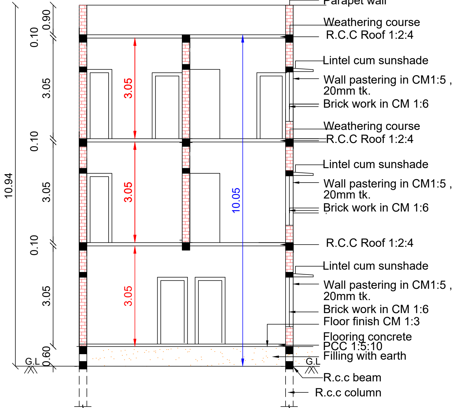
SECTION A-B
