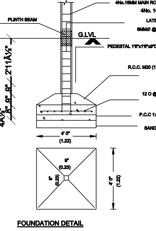
FOUNDAION DET.
