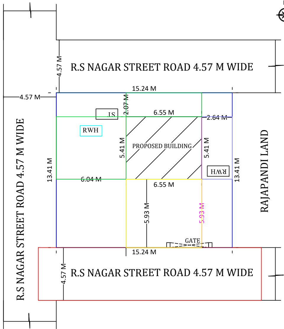
SITE PLAN 1:100 SCALE
