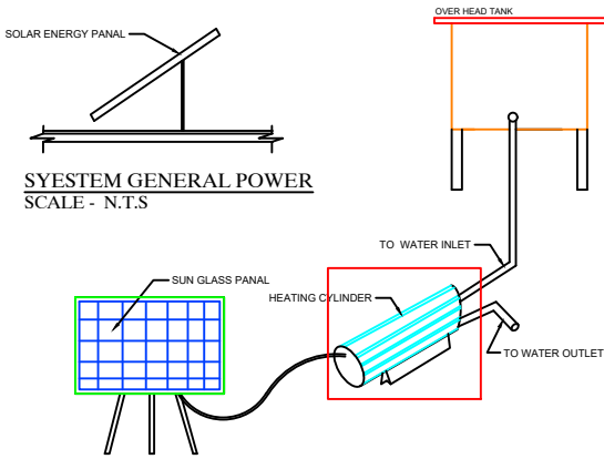
SOLAR WATER HEATING SYSETEM SCALE - N.T.S
