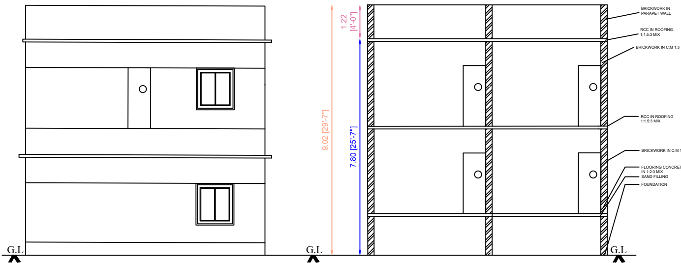
ELEVATION
