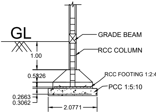
SECTION ON - BB (N.T.S.)
