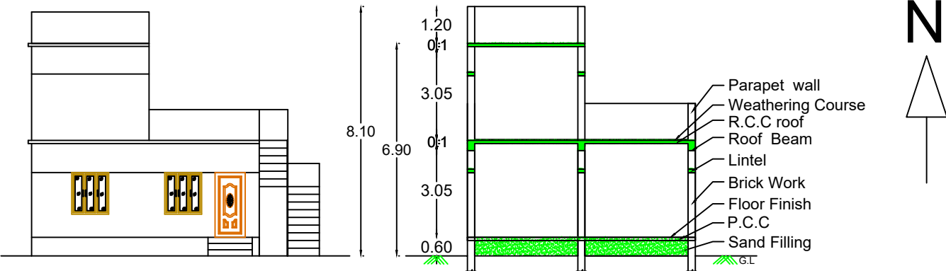
ELEVATION
