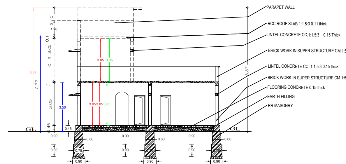
SECTION - 'A'-'B'
