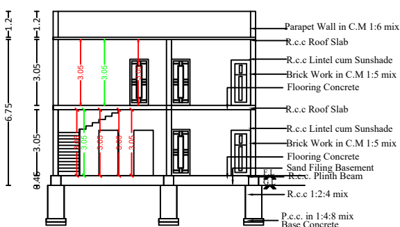
SECTION A-B
