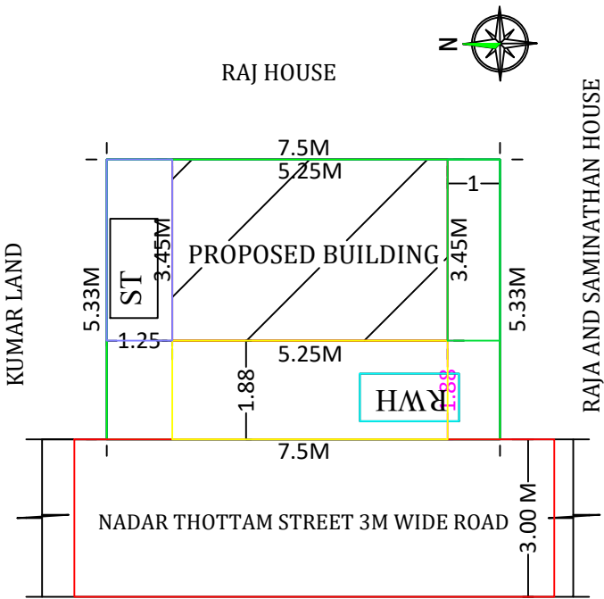
SITE PLAN 1:100 SCALE
