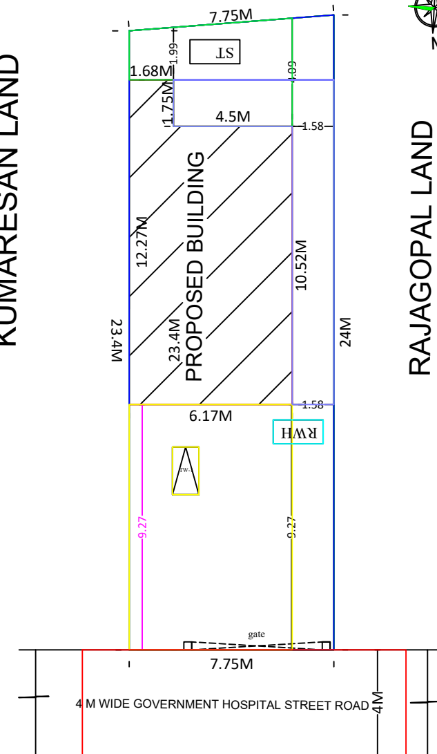
SITE PLAN 1:100 SCALE
