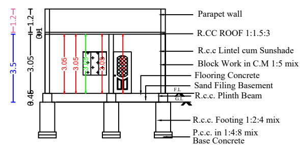
SECTION A-B
