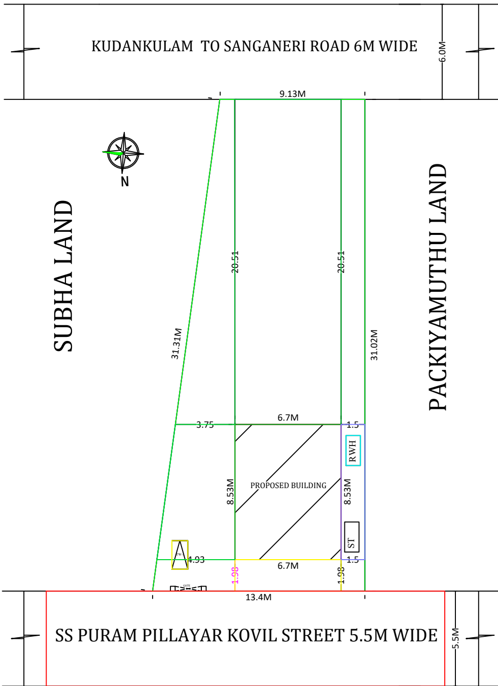
SITE PLAN 1:100 SCALE
