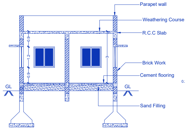
SECTION-A
