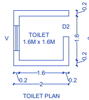
TOILET PLAN
