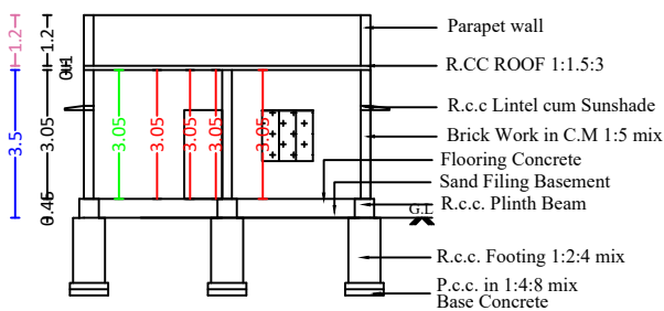
SECTION A-B
