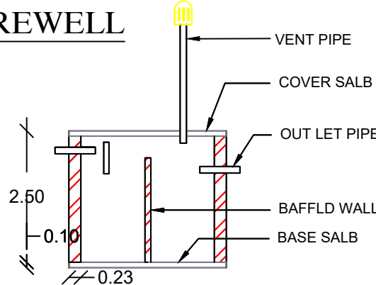
SECTION ON X - Y
