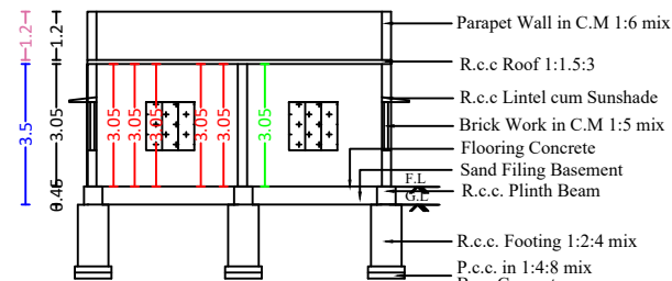
SECTION A-B
