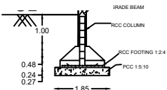
SECTION ON - BB (N.T.S)
