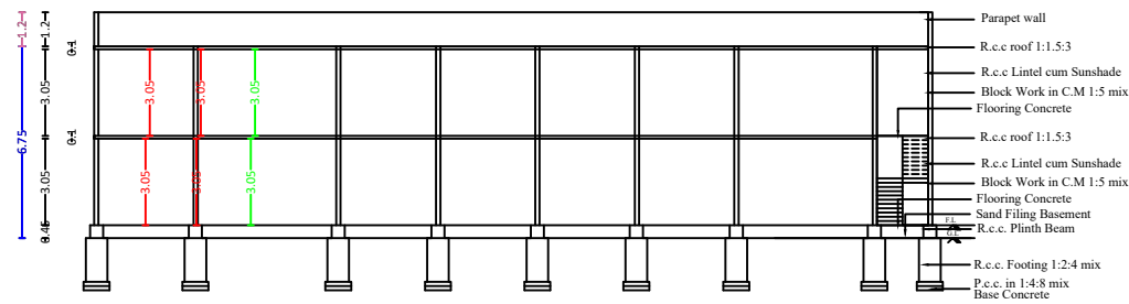
SECTION A-B
