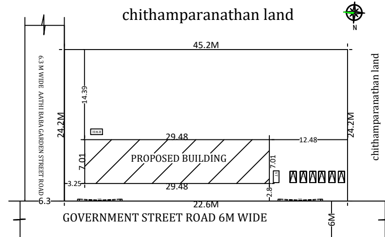
SITE PLAN 1:100 SCALE
