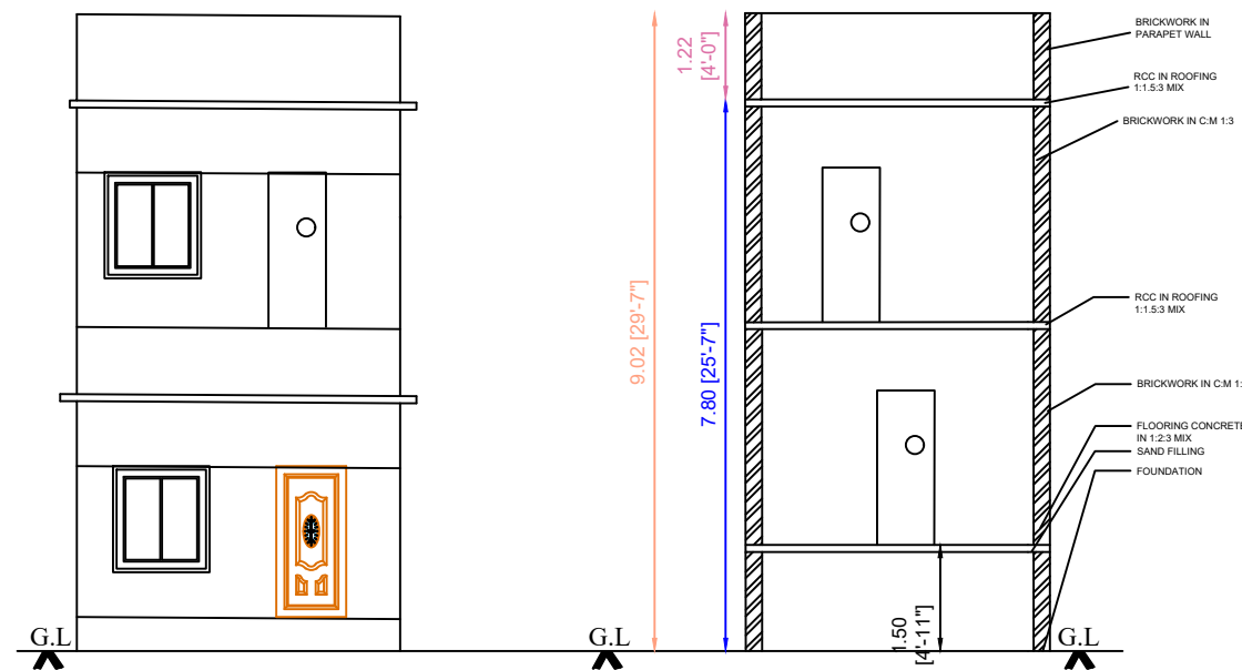
ELEVATION
